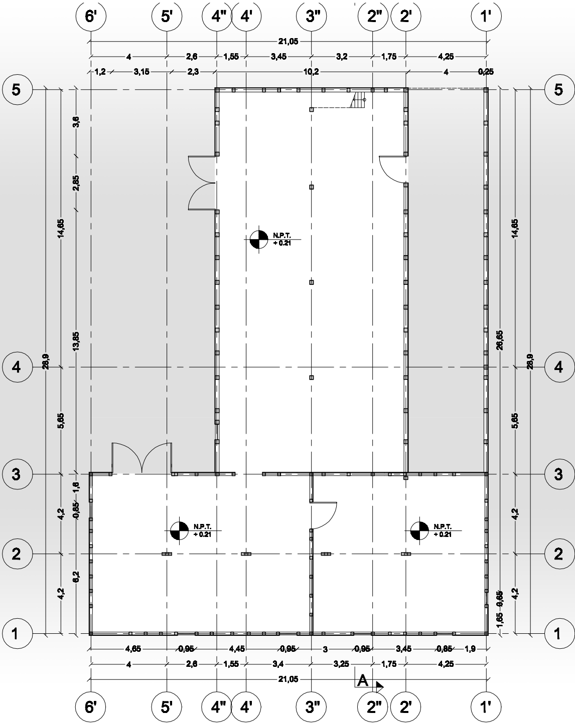
PLANTA SEGUNDO ESCALA 1/200
