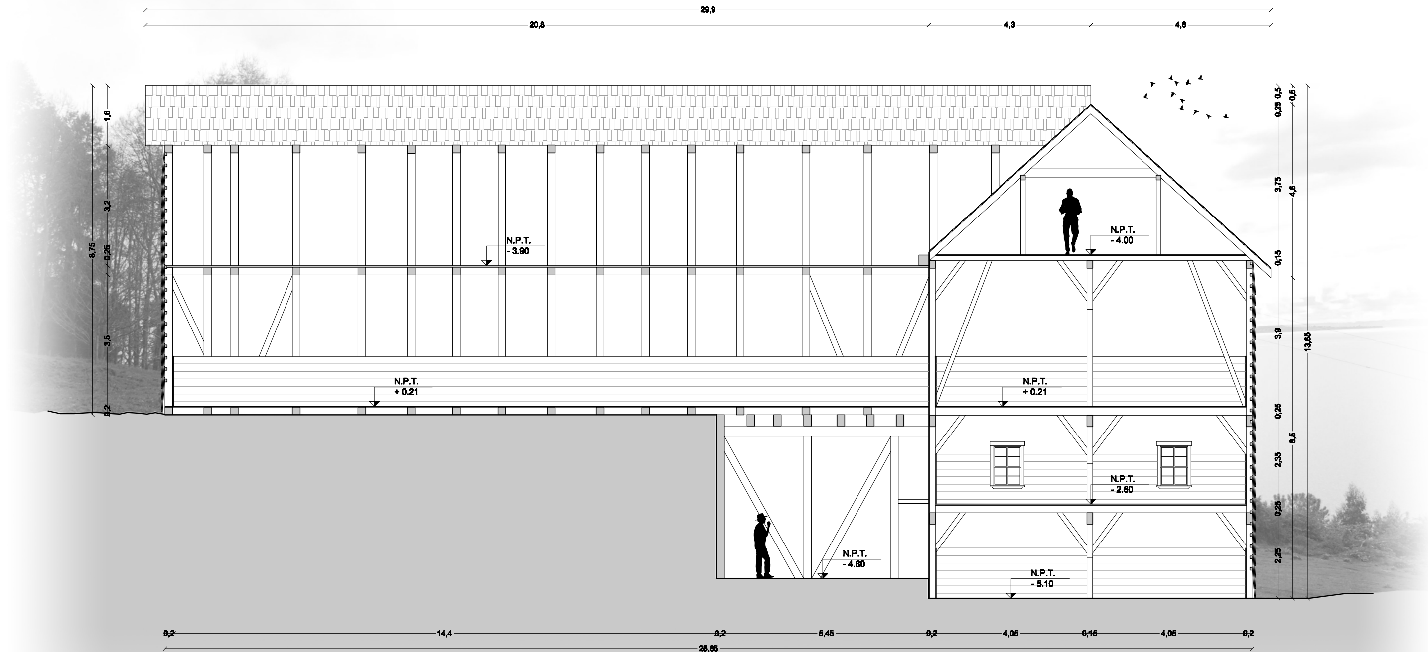
CORTE TRANSVERSAL A - A ESCALA 1/100
